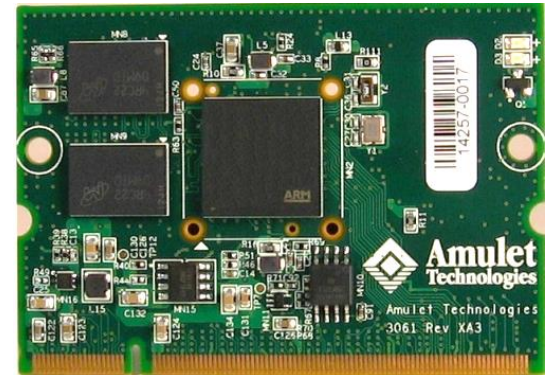
System-on-Module (SoM)
